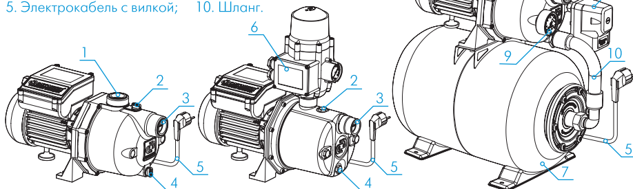
Поверхностный насос
