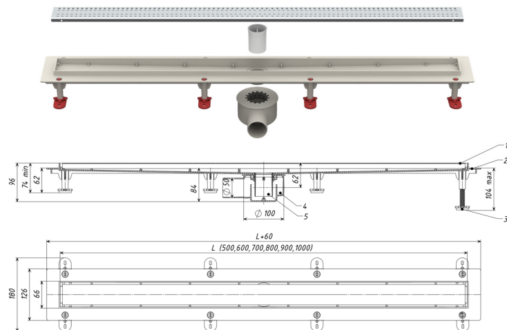
Рис. 1 – Габаритные размеры
