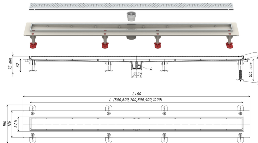
Рис. 1 – Габаритные размеры
