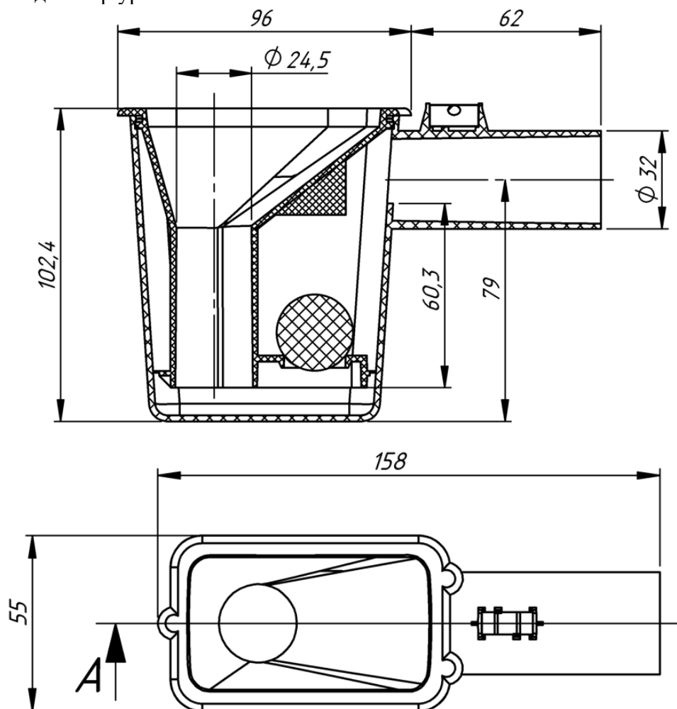
Рис. 1. Схема капельной воронки
