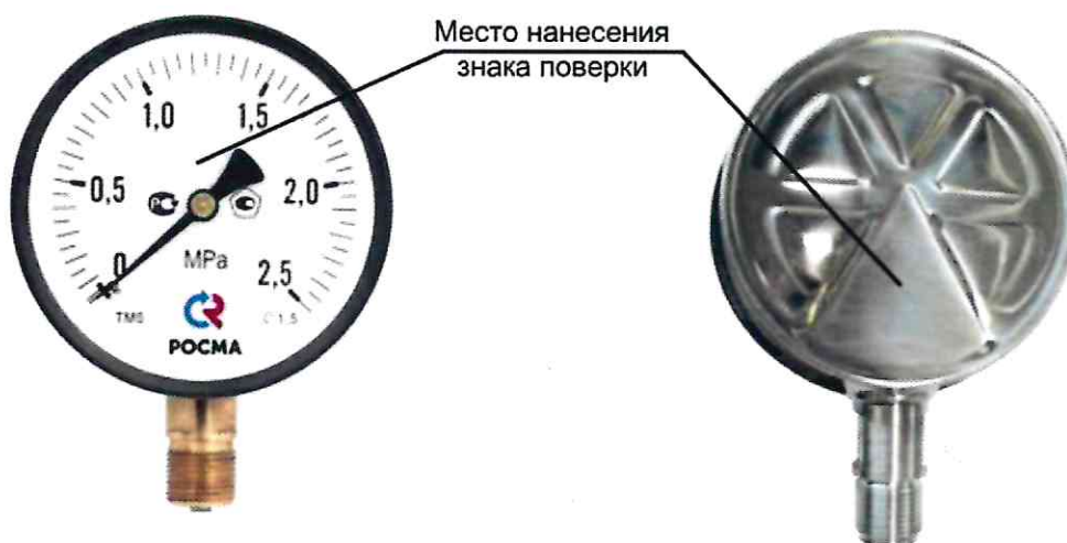
Рисунок 14 - Обозначение места нанесения знака поверки
