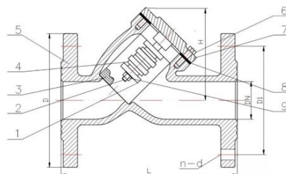
Рис.1 Фильтр сетчатый фланцевый.
